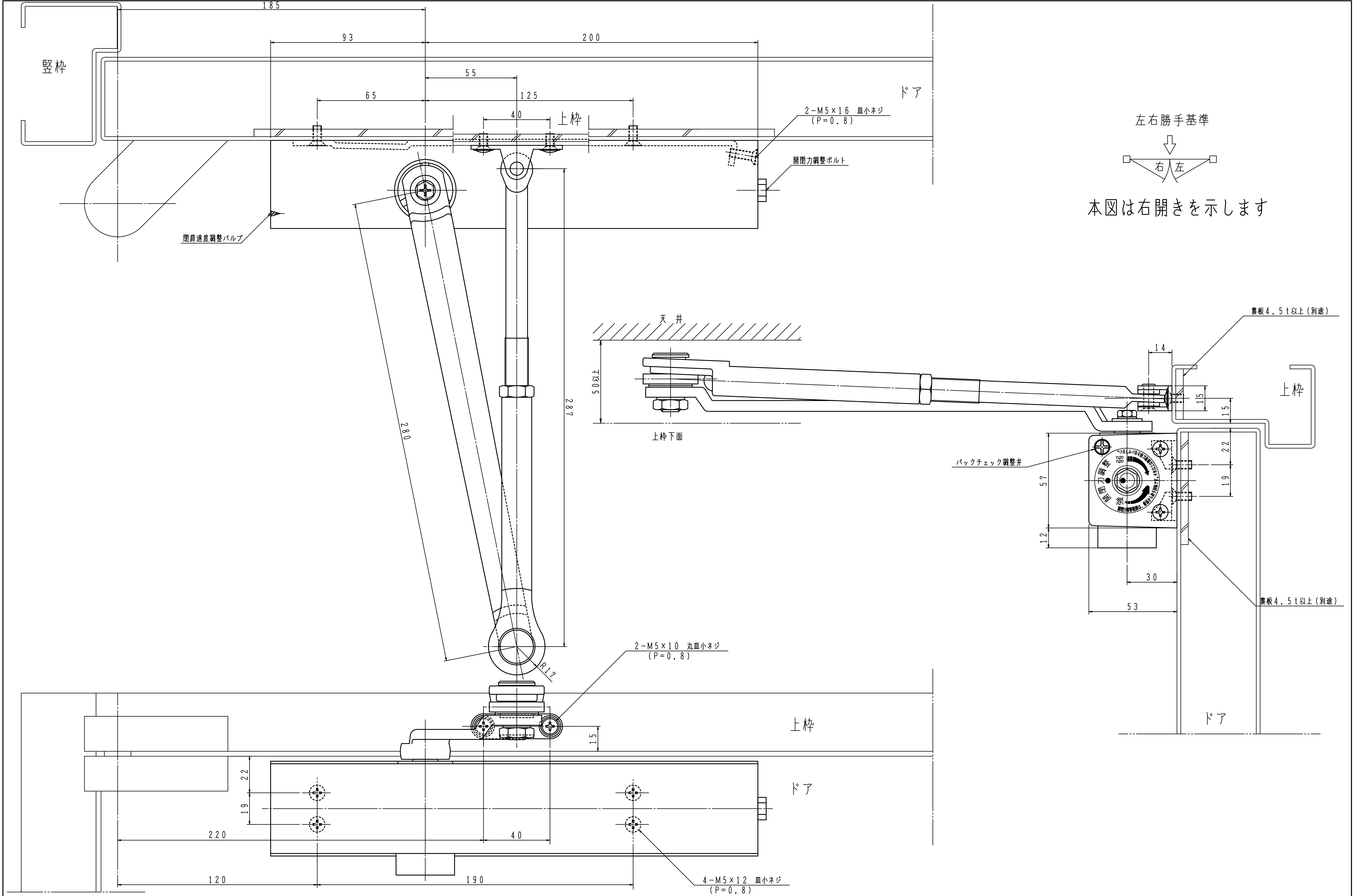
ドアクローザ S-7710V 納まり図
