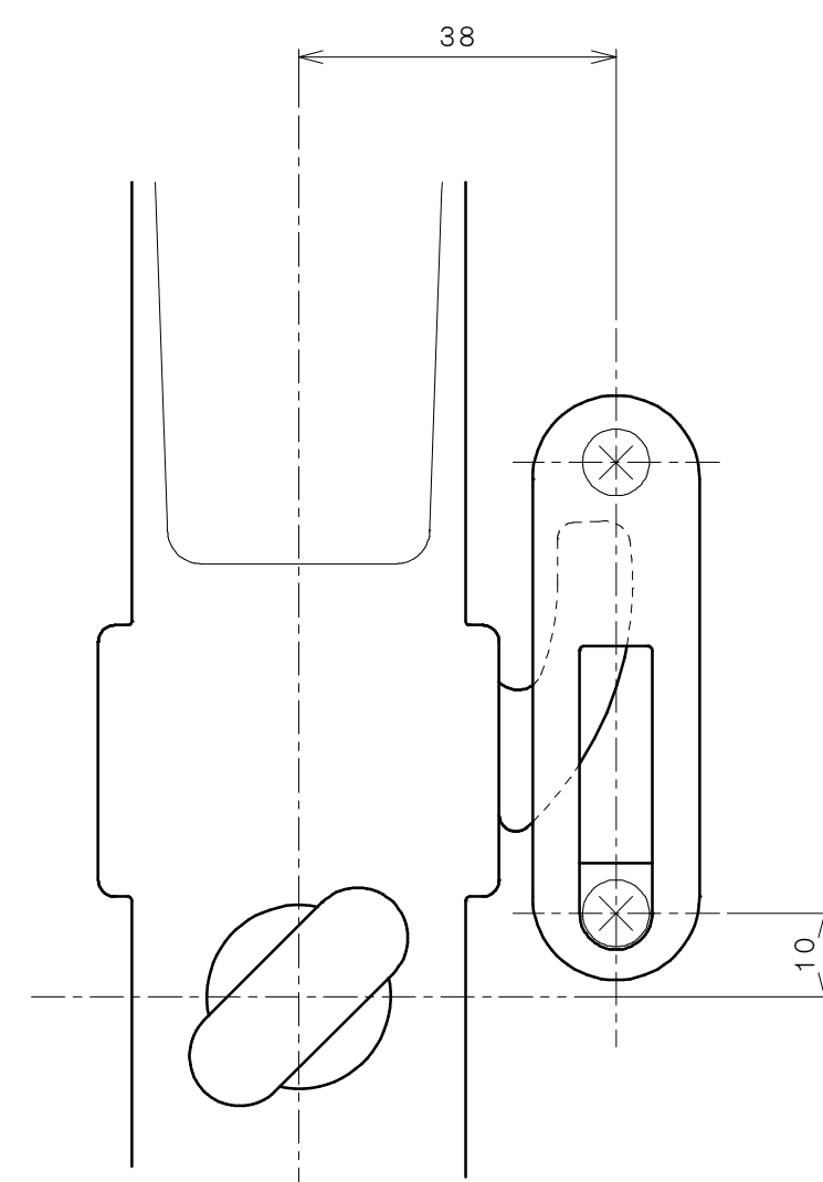
受箱 (A) 納まり図
