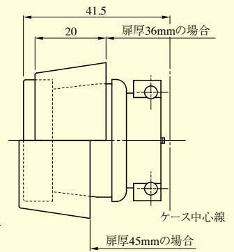
側面図（官民仕様）
