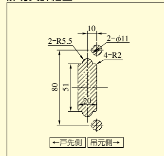
扉切欠詳細図
