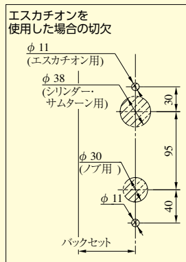
U型ノブ
