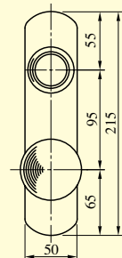
P型ノブ
