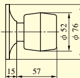
U型ノブ
