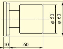
K型ノブ
