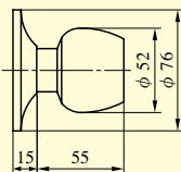
W型ノブ
