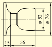
D型ノブ
