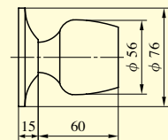
P型ノブ
