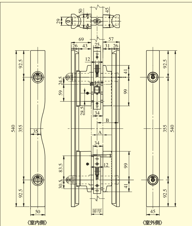
【外形寸法図】
