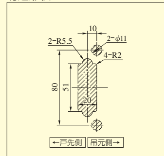
切込形状
