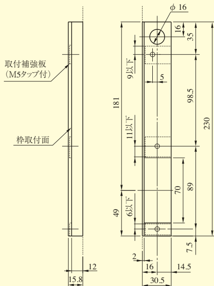
枠側の切欠寸法
