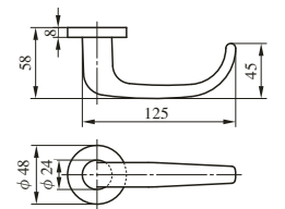
ZLK980型
