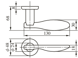
ZLK96402型
