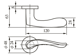
ZLT902型
