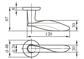
ZLK95402型
