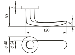
ZLT901型
