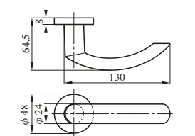
ZLK983型
