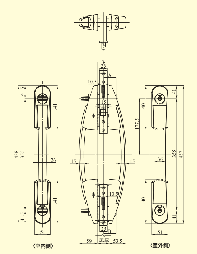
【外形寸法図】 PRPGF713W-1型
