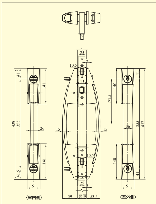
【外形寸法図】 PRPGF714W-1型
