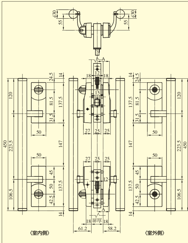
【外形寸法図】 PRPGVF571DV-1型
