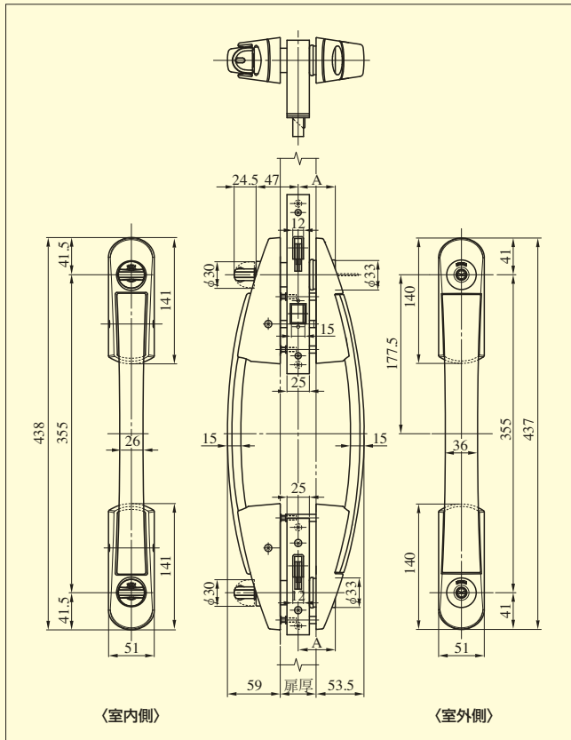
【外形寸法図】 PRPGVF713W-1型
