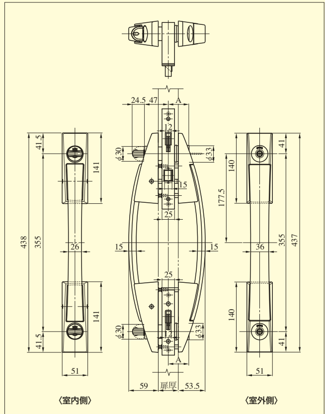
【外形寸法図】 PRPGVF714W-1型
