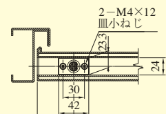
下部ロッドガイド正面図
