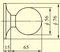
Q型ノブ
