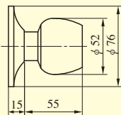
K型ノブ
