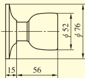
Q型ノブ
