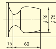
P型ノブ
