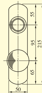
P型ノブ
