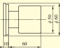
K型ノブ
