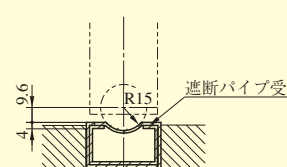
遮断パイプ受図 (お客様御手配品)
