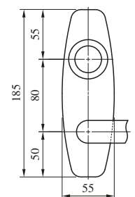
黄銅ヘアライン (BS)
