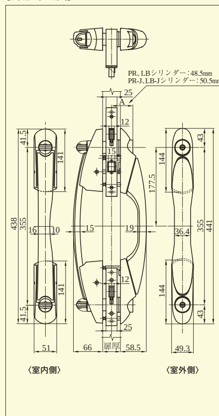
【外形寸法図】 U9PGVF705DV-1 型
