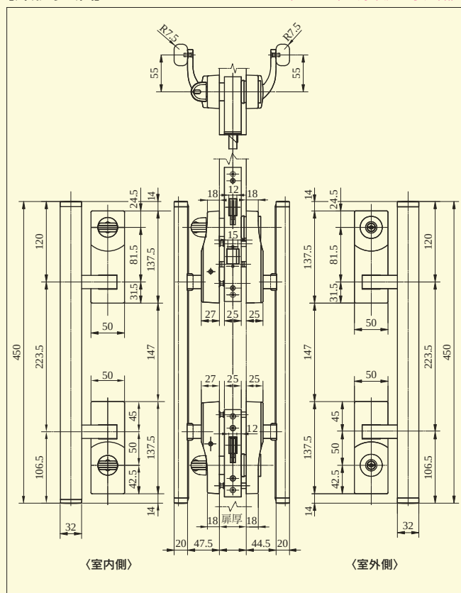
【外形寸法図】 U9PGVF572DV-1 型 (2011年3月末廃止予定品)
