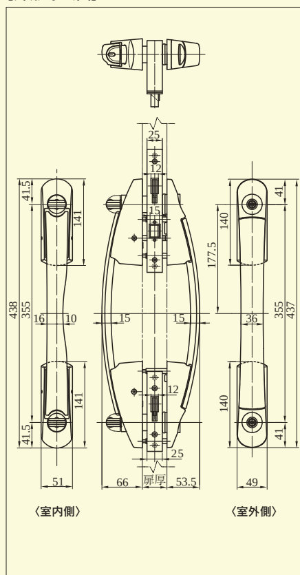
【外形寸法図】 U9PGVF703DV-1 型
