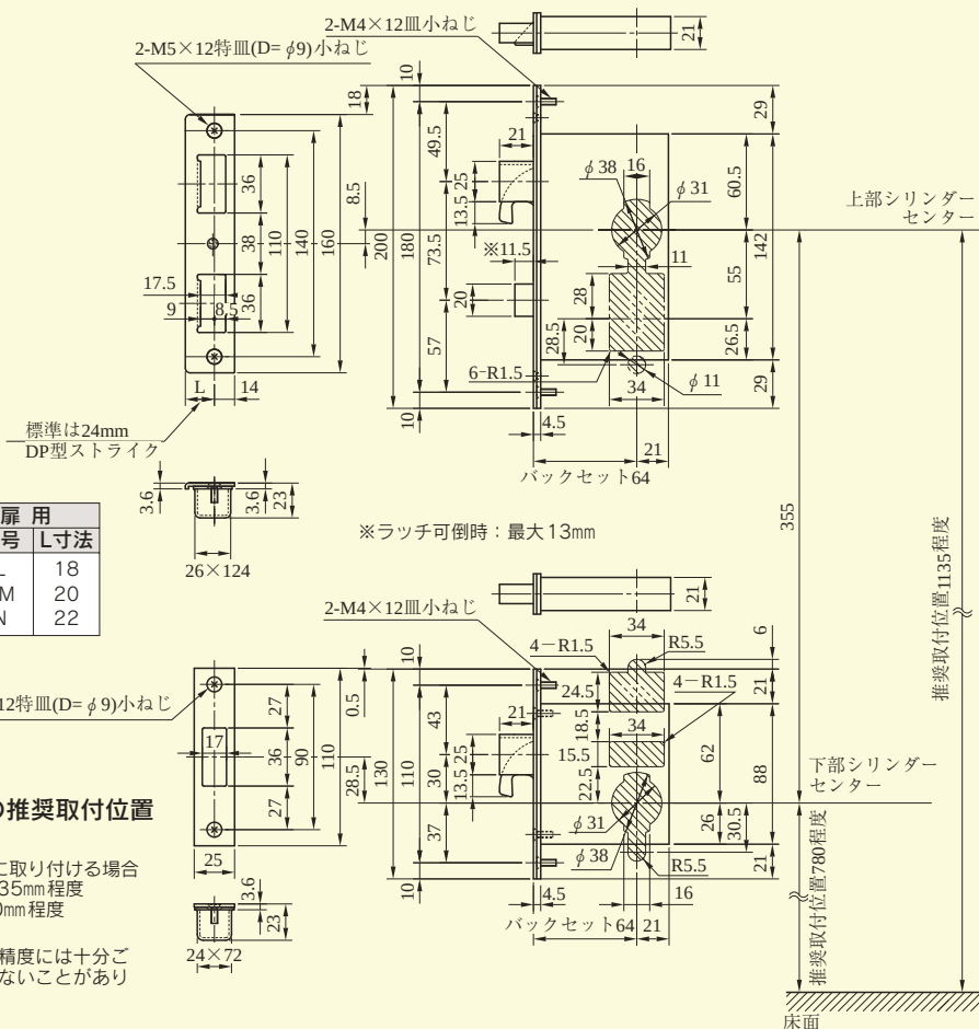
【外形寸法図】 PRPGF704DW-1 型
