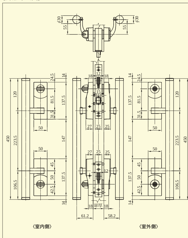
【外形寸法図】 U9PGVF571DV-1 型
