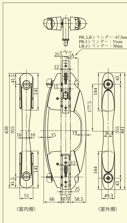
【外形寸法図】 PRPGF705DW-1 型
