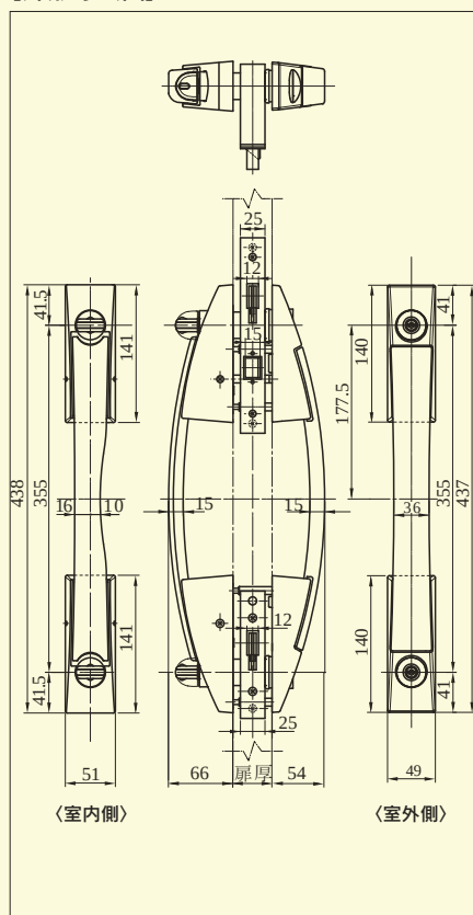
【外形寸法図】 U9PGVF704DV-1 型
