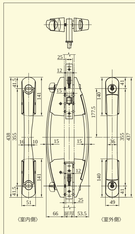
【外形寸法図】 PRPGF703DW-1 型
