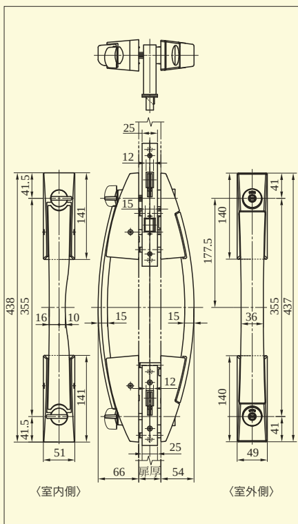
【外形寸法図】 PRPGF704DW-1 型
