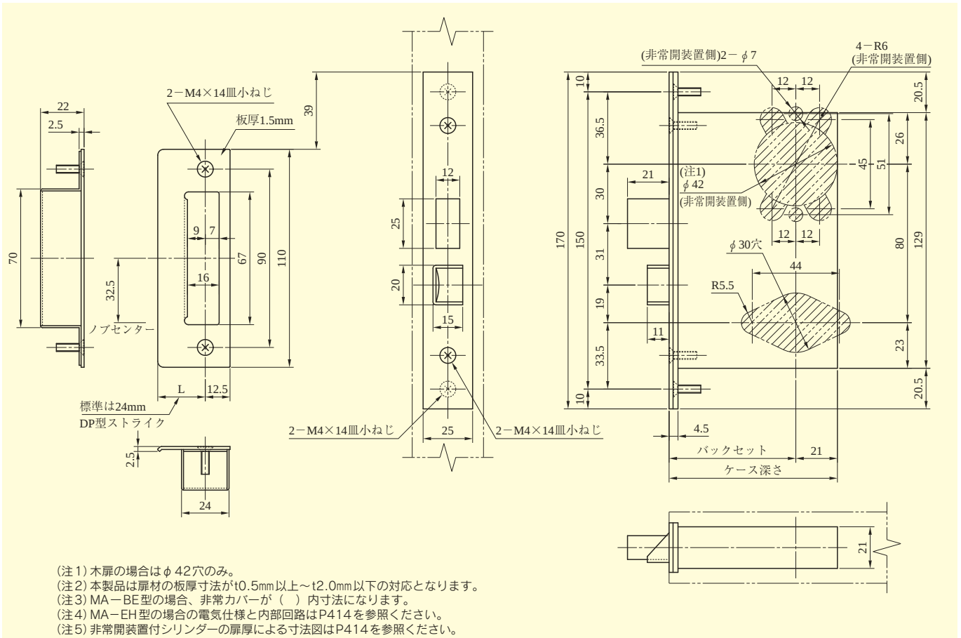
●扉厚によるストライクのL寸法(単位mm)
