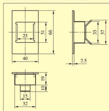
扉切込加工参考図
