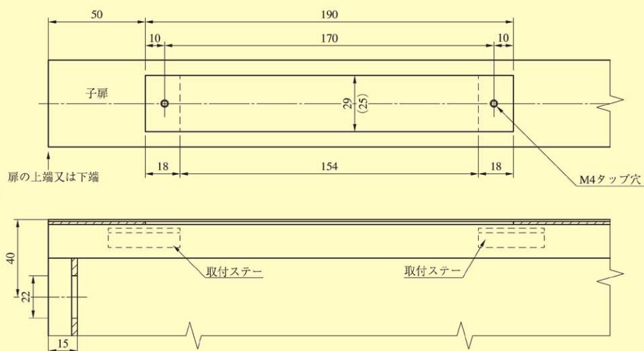
扉切込加工参考図
