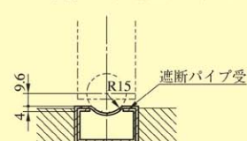
遮断パイプ受図(客先ご手配品)
