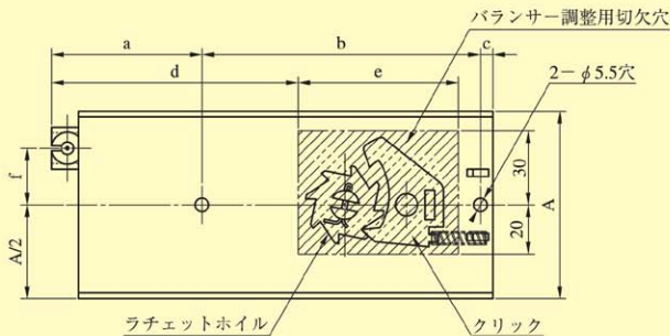
バランサー(単装)
