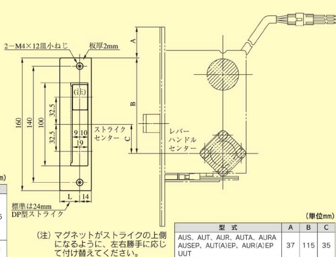
N1-01AM・STB型
