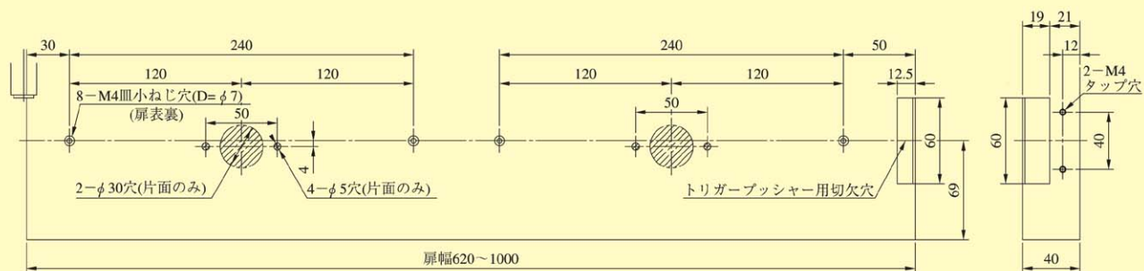
XS2B型扉切欠図
