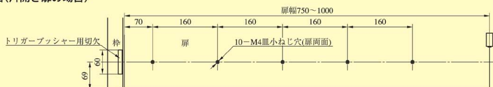
XSA型扉、枠切欠図(片開き扉の場合)
