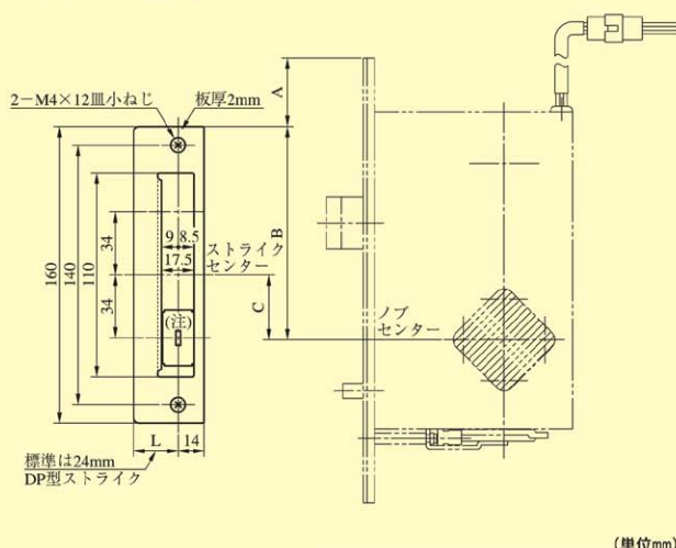
N1-01AM・STB型
