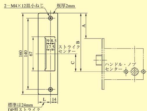
N1-02・STB型
