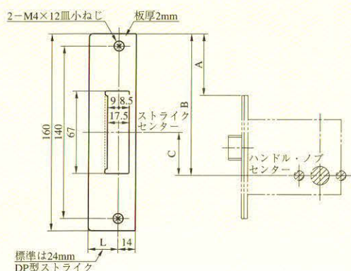
N1-02・STB型
