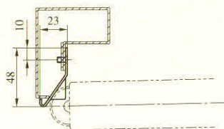
トリガープッシャー取付図
