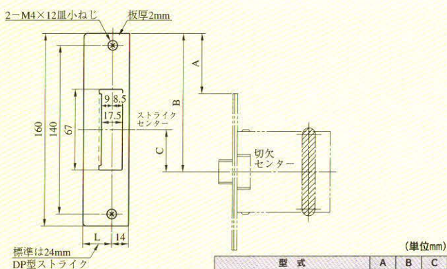
N1-02・STB型(OPJ(S)の場合)
