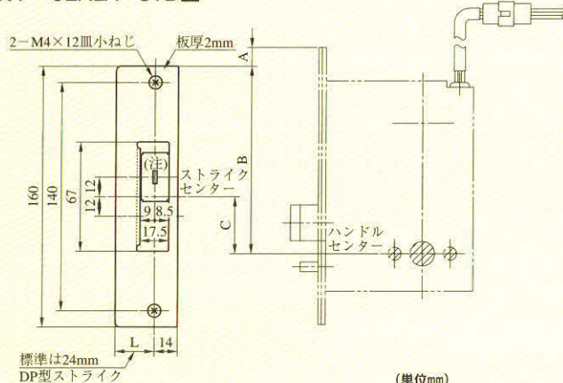
N1-02ALA・STB型
