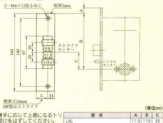
N1-02LAL・STB型
