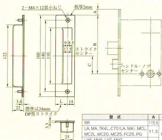
N1-01・STB型
