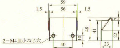
トリガープッシャー外形図
