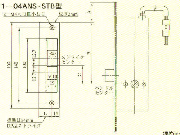
N1-04ANS・STB型
