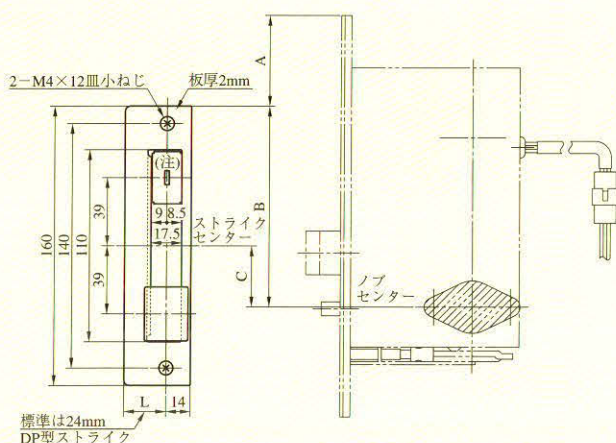
N1-01AL・STB型
