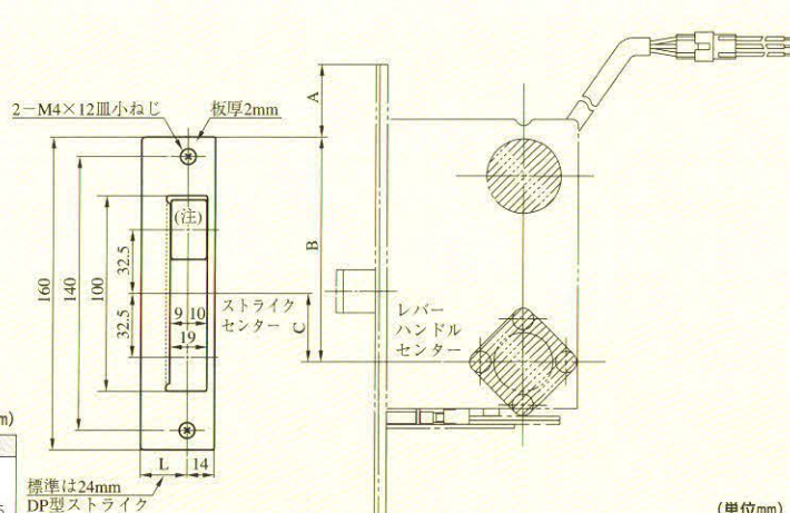
N1-04AU・STB型
