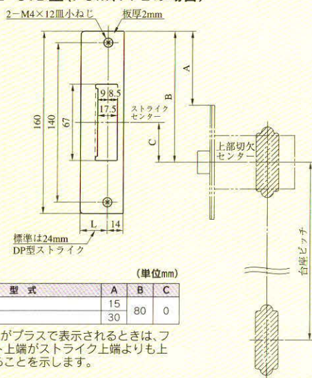
N1-02・STB型(POM、PPLの場合)
