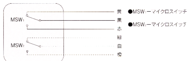
(本図はキースイッチOFF位置を示す) 破線は、KS-110W、KS-220Wシリーズを示す
