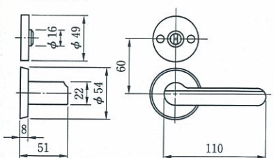
●外観寸法図
