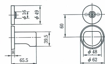
● 外観寸法図
