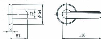
●外観寸法図
