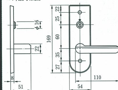
●外観寸法図
