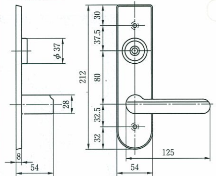
●外観寸法図
