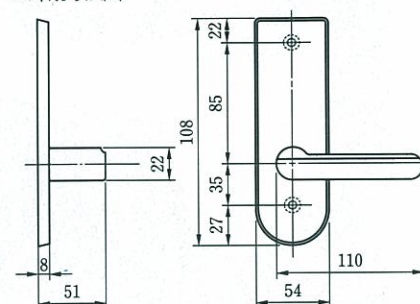
●外観寸法図
