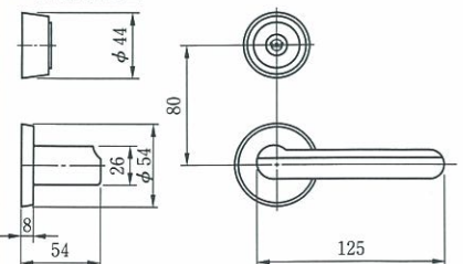
●外観寸法図
