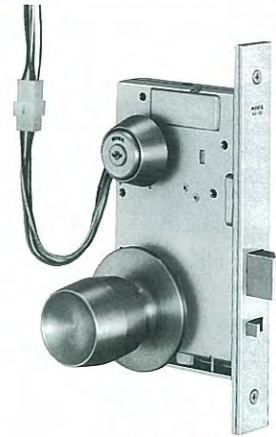
電気錠・ALシリーズ
