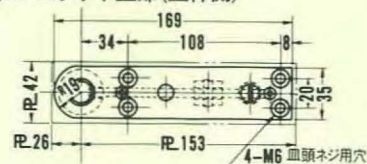
■トップピボット上部(上枠側)
