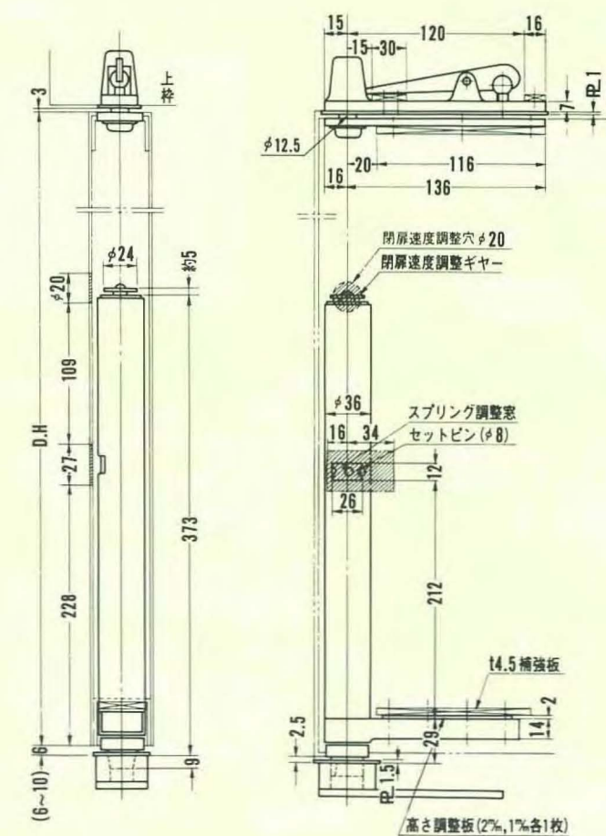
■ドア側
