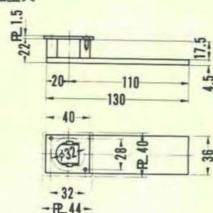
■埋込金具
