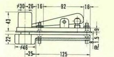
■トップピボット下部(ドア側) 4-M6 皿頭ネジ用穴
