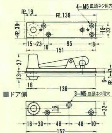
■埋込金具
