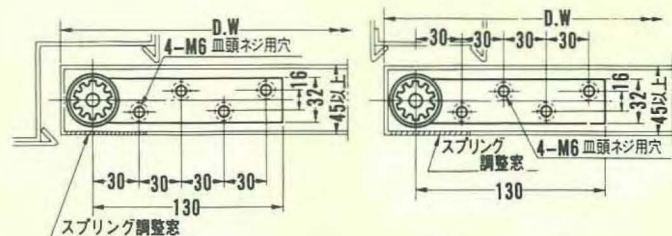
■90°開きの場合
