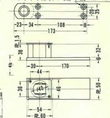
■トップピボット下部(ドア側) 4-M6 皿頭ネジ用穴
