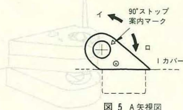
図 5 A 矢視図
