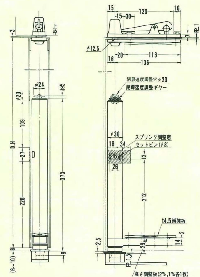
■ ドア側
