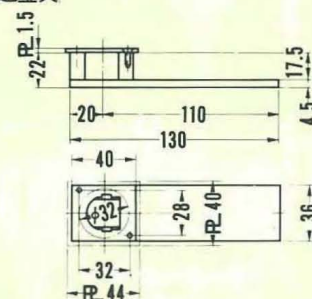
■埋込金具
