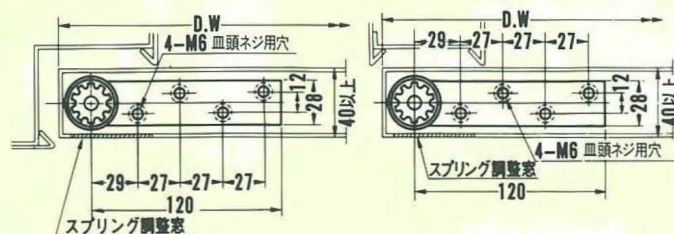
■90°開きの場合
