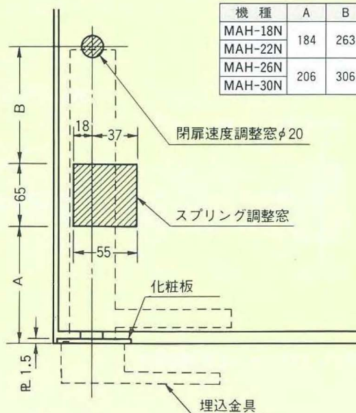
扉切欠き寸法図(単位mm)
