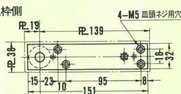
■上枠側
