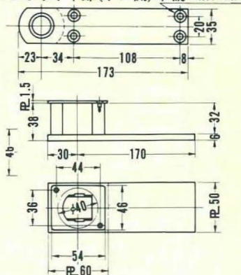
■トップピボット下部(ドア側) 4-M6 皿頭ネジ用穴
