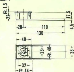
■埋込金具
