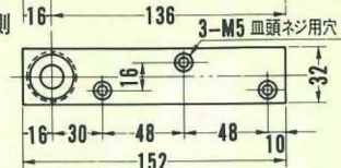
■埋込金具
