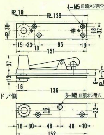
■埋込金具
