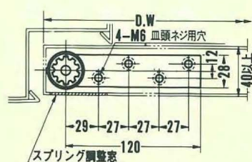
■90°開きの場合
