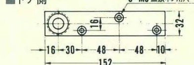
■埋込金具
