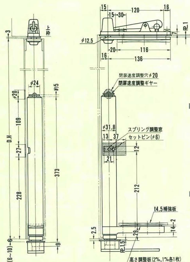
■埋込金具
