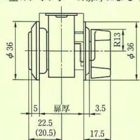
SL77-1型のシリンダーの扉厚による寸法図
