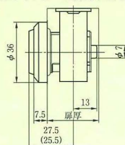
SL77-2型のシリンダーの扉厚による寸法
