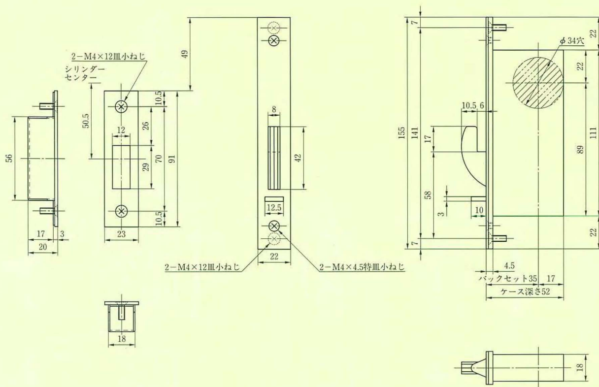
シリンダーの扉厚による寸法図
