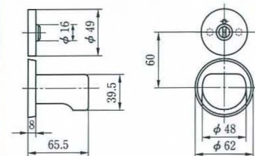
●外観寸法図
