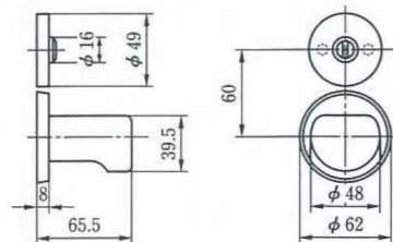
●外觀寸法図
