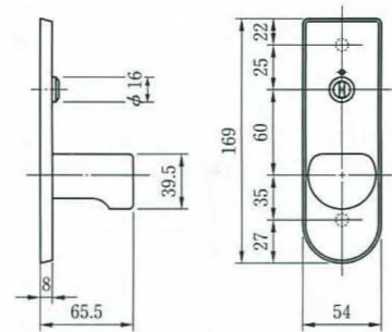
●外觀寸法図
