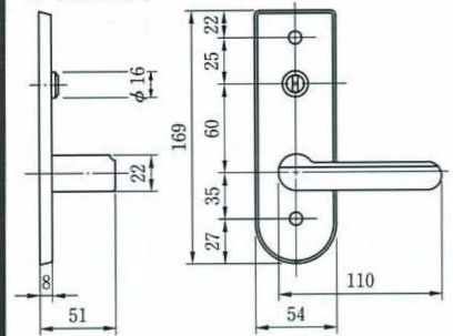
●外観寸法図
