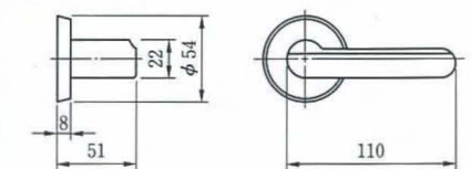
●外観寸法図
