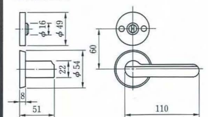
●外観寸法図
