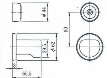
●外観寸法図
