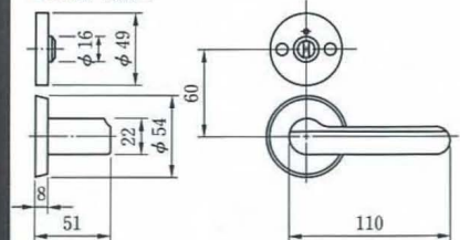
●外観寸法図
