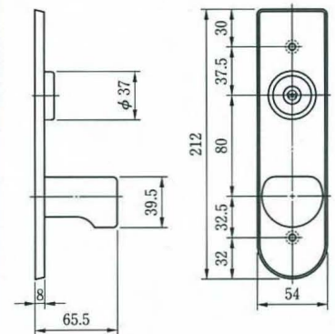
●外観寸法図
