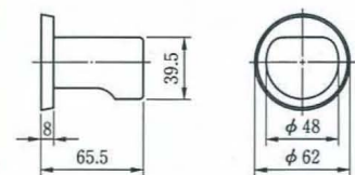
●外觀寸法図
