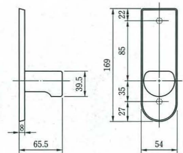
●外觀寸法図
