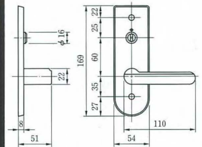
●外観寸法図
