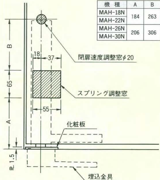
扉切欠き寸法図(単位mm)
