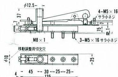
U型トップピボット
