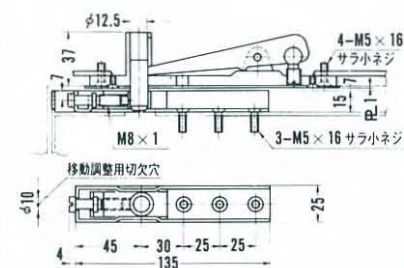
U型トップヒボット
