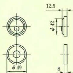
01型丸座+シリンダー、サムターン
