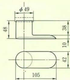
04型レバーハンドル
