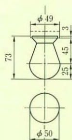
54型ノブ
