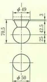
53型ノブ
