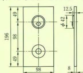
11型エスカチオン+シリンダー、サムターン
