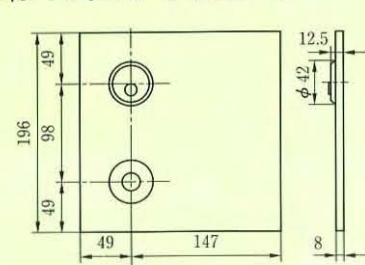
12型エスカチオン+シリンダー、サムターン
