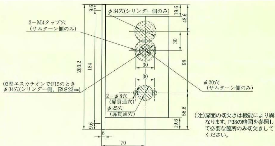
01型丸座、03型エスカチオン用切込外観図
