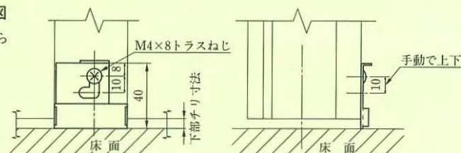
XSB型遮断ピース召合せ部取付図
