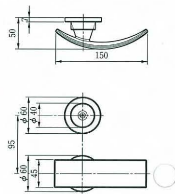
●外観寸法図
