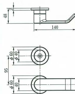
●外観寸法図
