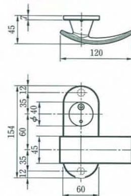
●外観寸法図
