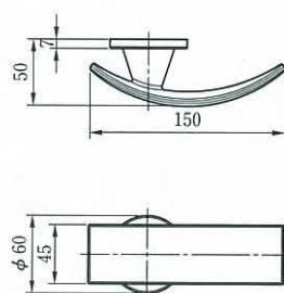
●外観寸法図
