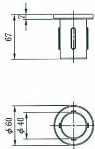
●外観寸法図
