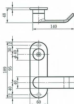
●外観寸法図
