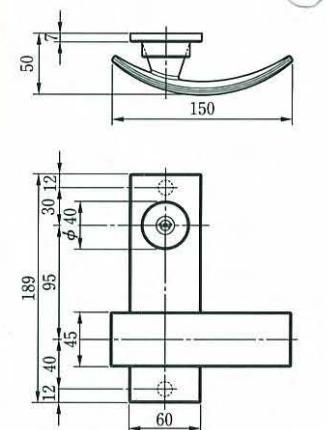
●外観寸法図
