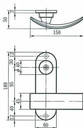
●外観寸法図
