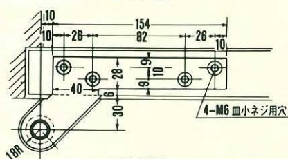
■上枠側
