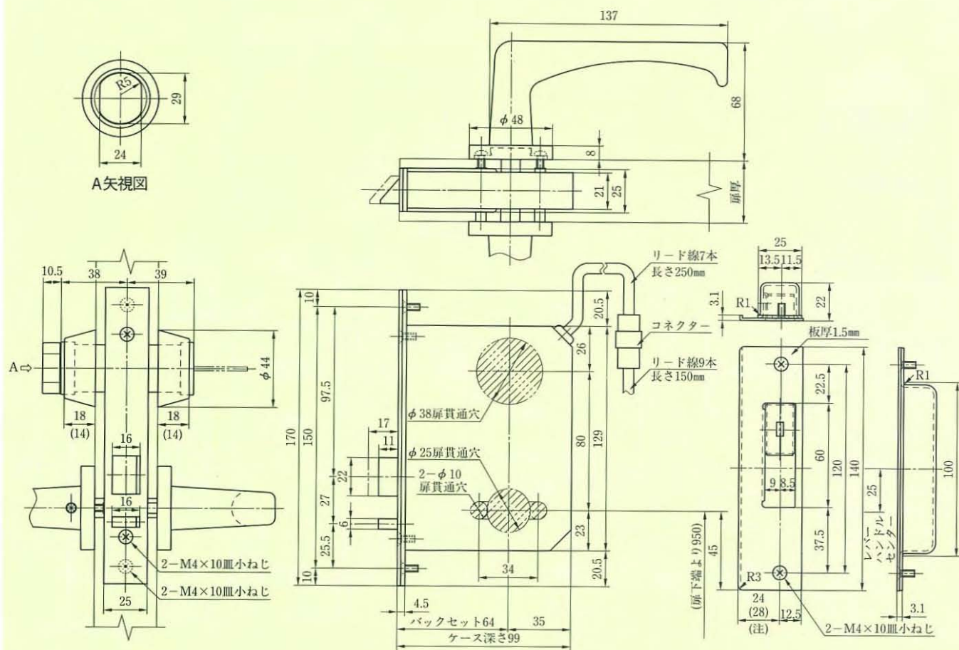
ALX-BL型(7線式)
