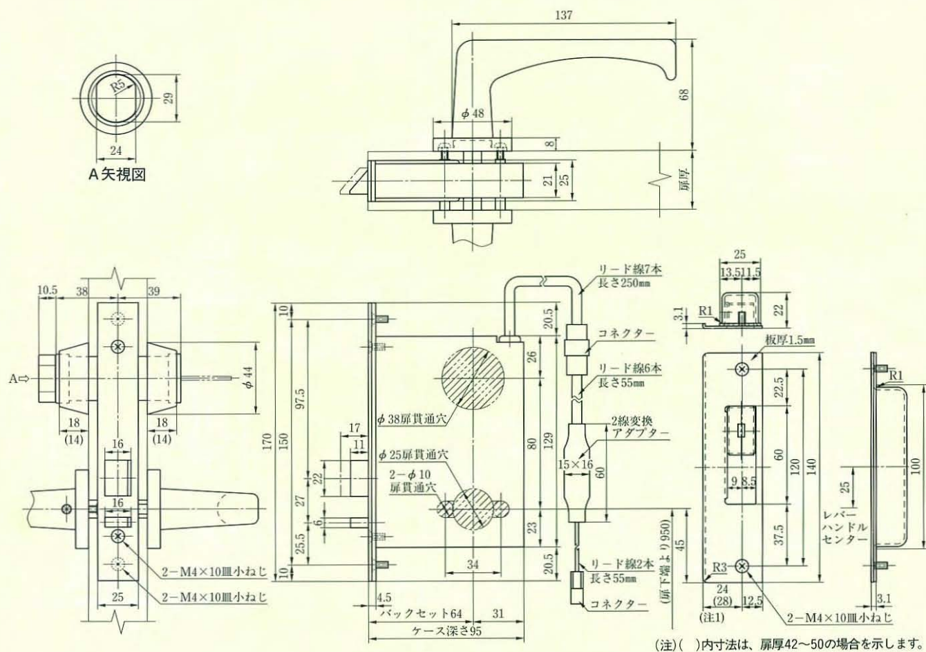
20ALA-BL型(2線式)
