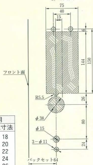
扉切欠図
