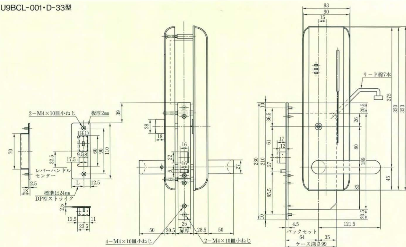
扉切欠図
