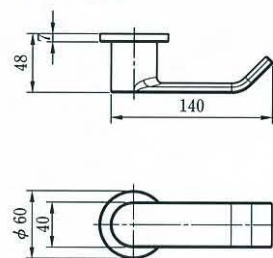
●外観寸法図
