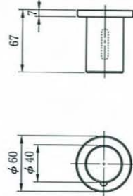
●外観寸法図
