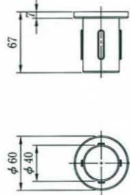
●外観寸法図
