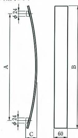
●外観寸法図
