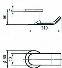
●外観寸法図
