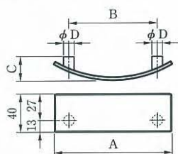
●外観寸法図
