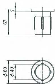
●外観寸法図
