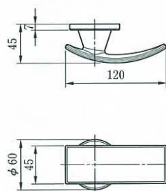
●外観寸法図
