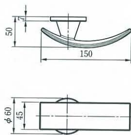
●外観寸法図
