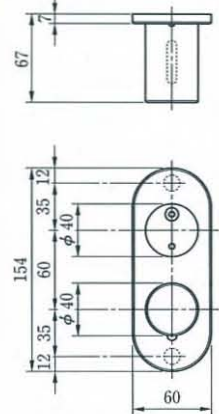
●外観寸法図
