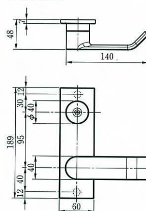
●外観寸法図
