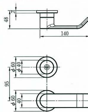
●外観寸法図
