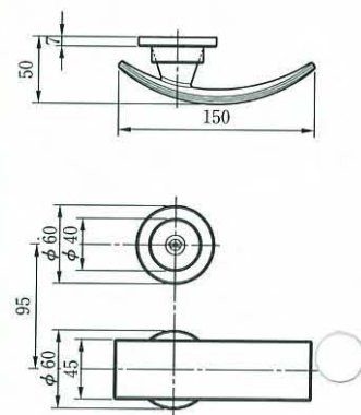
●外観寸法図
