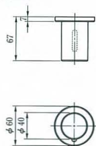
●外観寸法図
