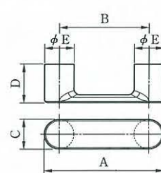
●外観寸法図
