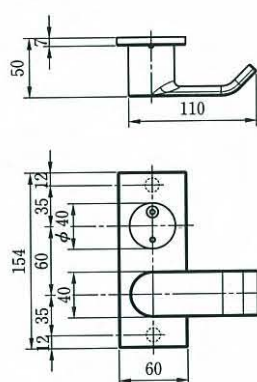
●外観寸法図
