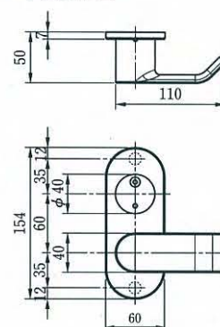
●外観寸法図
