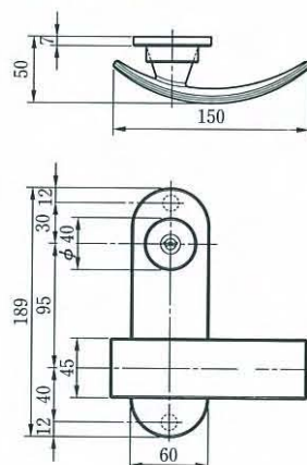
●外観寸法図
