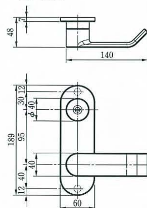
●外観寸法図
