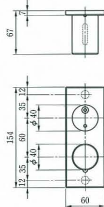
●外観寸法図
