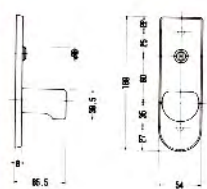
■H70130 ■H70105 影込引手
