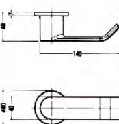
■ LG1214-8 表示付非常開装置錠
