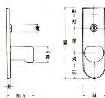
■T70108 ■T70093 ■T70078 ■T70063 取手
