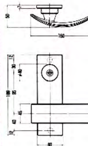
■ LG1213-8 表示付非常開装置錠
