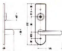
■ LG7676-8 表示付非常開装置錠
