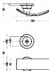
■ U9LHS1314-1 シリンダー錠
