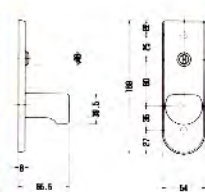
■H70130 ■H70105 彫込引手
