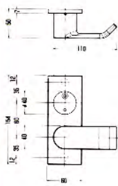
■ U9MHS1710-1 シリンダー錠
