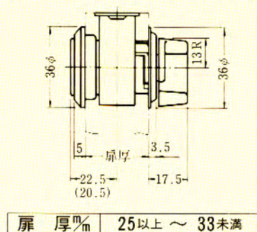
SL77-1型のシリンダーの扉厚による寸法図
