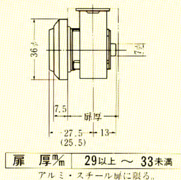
SL77-2型のシリンダーの扉厚による寸法図
