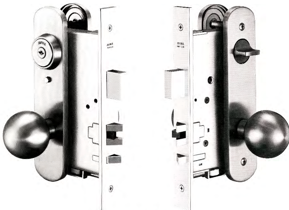
U9MHHQ型 (内開き右勝手を示す)
