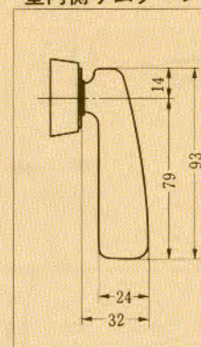
室内側サムターン
