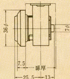
SL77-2型のシリンダーの扉厚による寸法図
