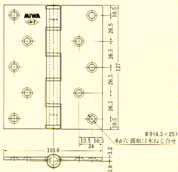
127×102型
