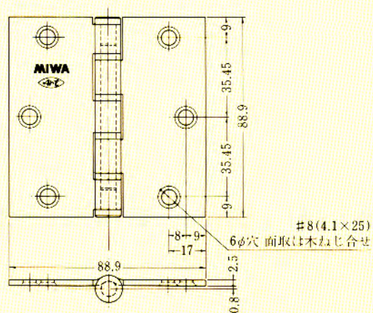
89型
