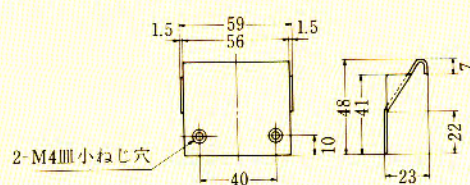
トリガープッシャー外形図
