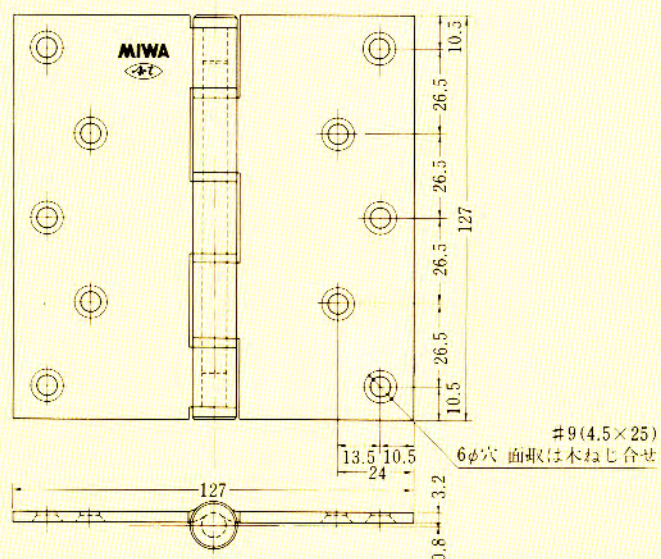
127型
