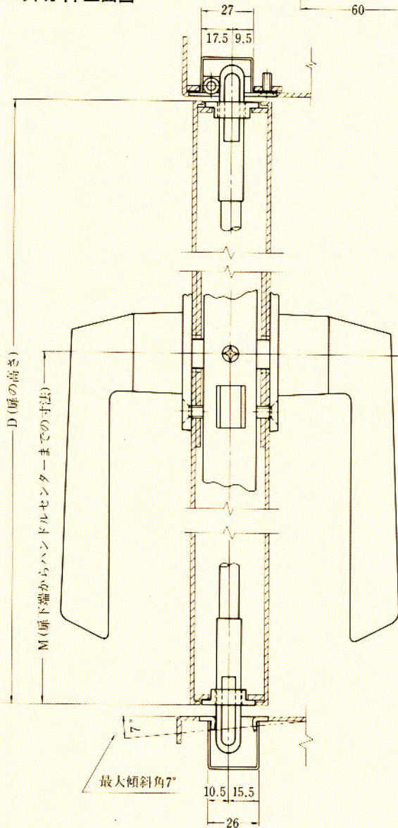
ロッドガイド正面図
