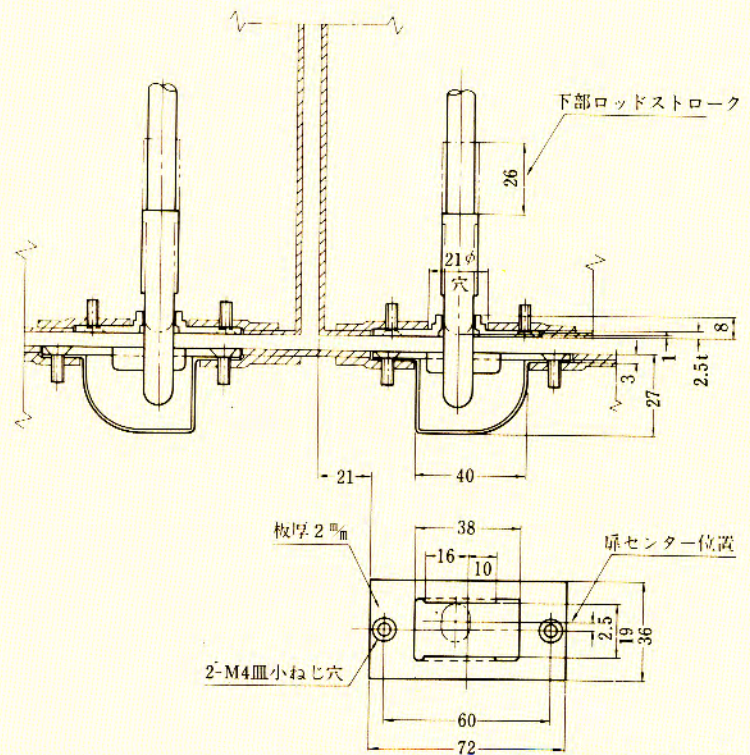
下部受正面図
