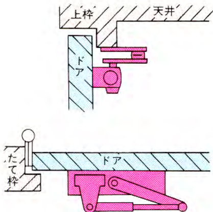
基準図
