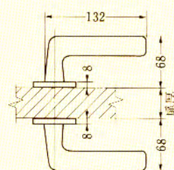
52型ハンドル
