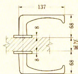
50型ハンドル
