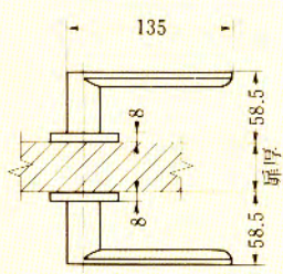
66型ハンドル
