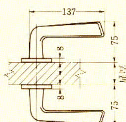
51型ハンドル
