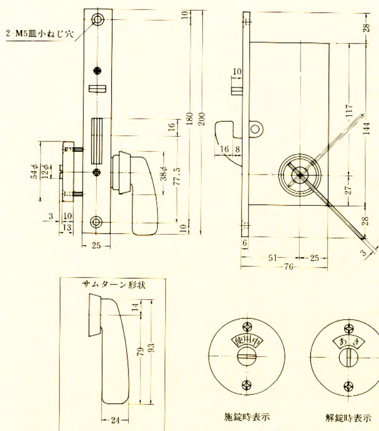
●2FD-EI型切込外観図
