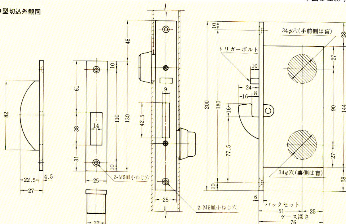
●2FD-EI型切込外観図
