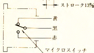
BH-EPK・H信号回路 (本図は解錠時を示す)
