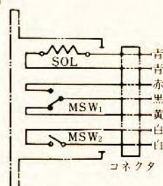
内部回路図
