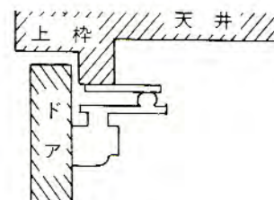
基準図
